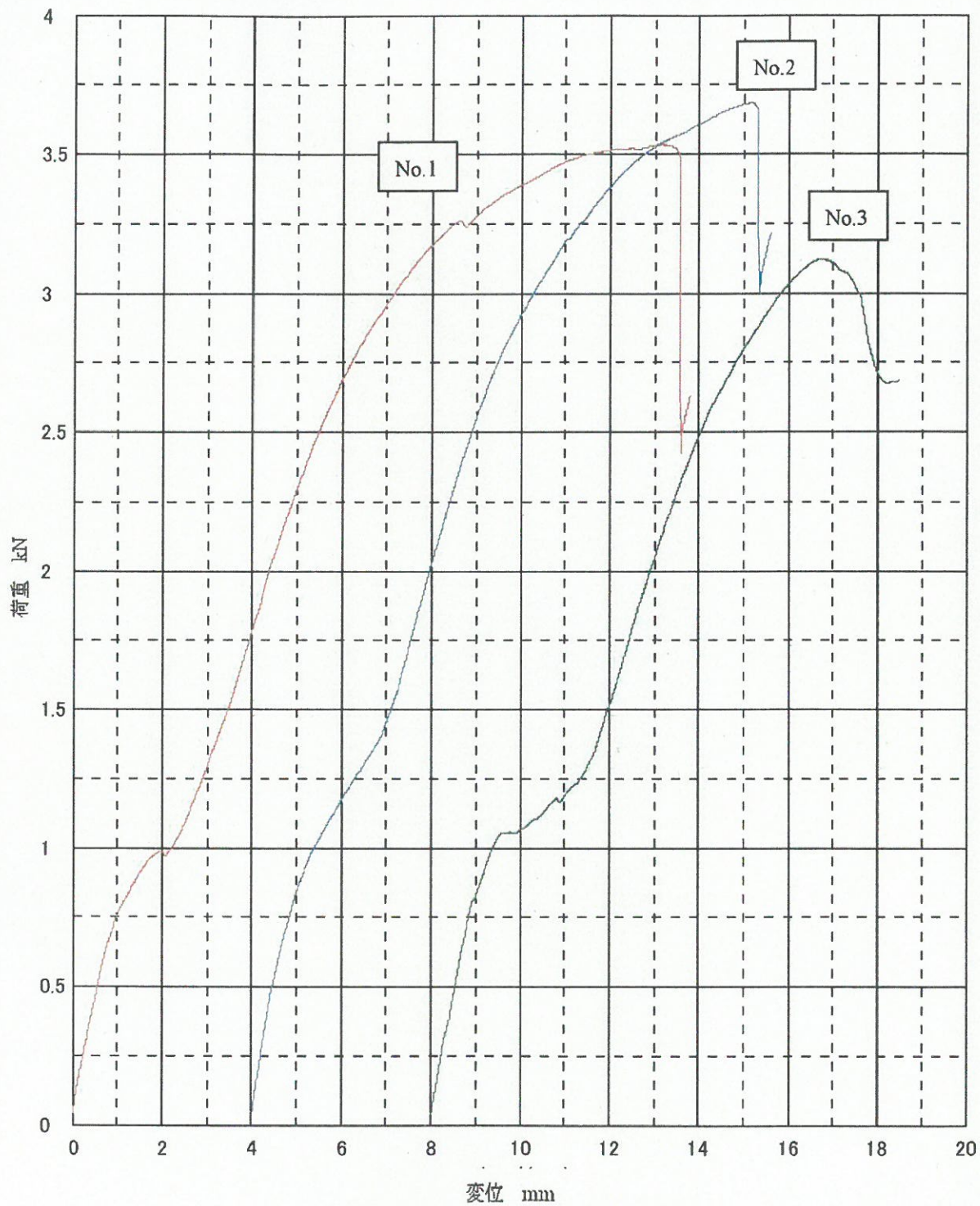
第H24456号 別紙：荷重—変位線図
