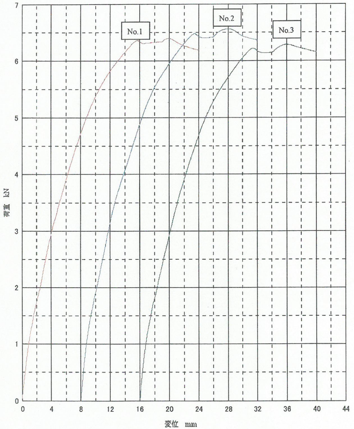
第H24456号の2 別紙：荷重—変位線図
