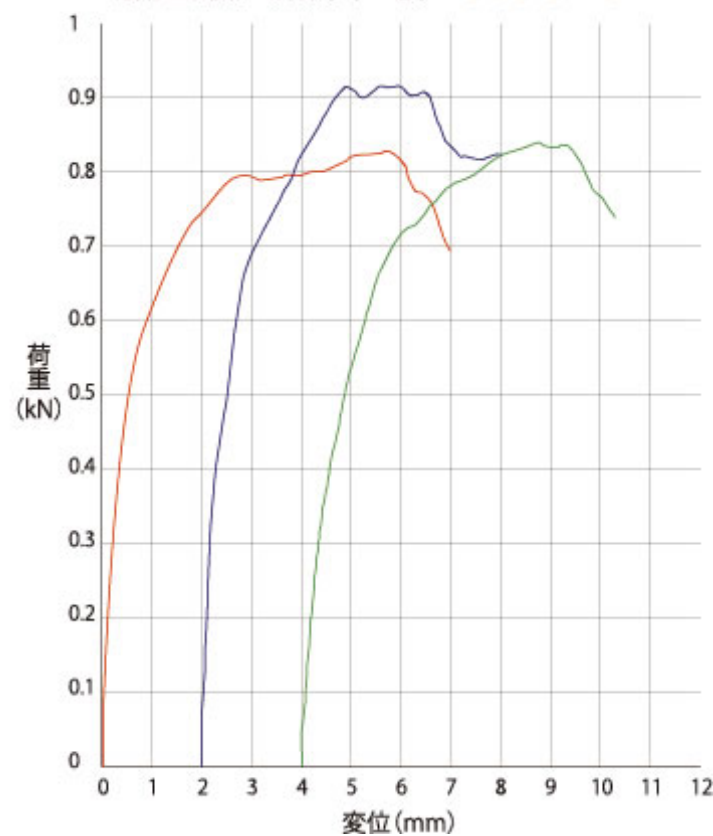
【③ハゼ取付金具滑り試験(単体)】
