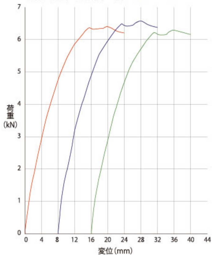
【②ハゼ取付金具圧縮試験(単体)】
